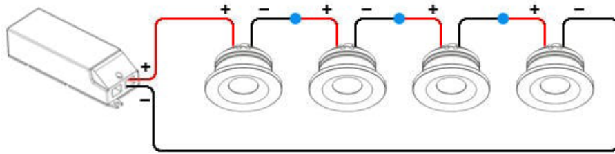
चित्र 2.3.1(ए) 350mA, 500mA, 700mA, और 1050mA पर श्रृंखला कनेक्शन
