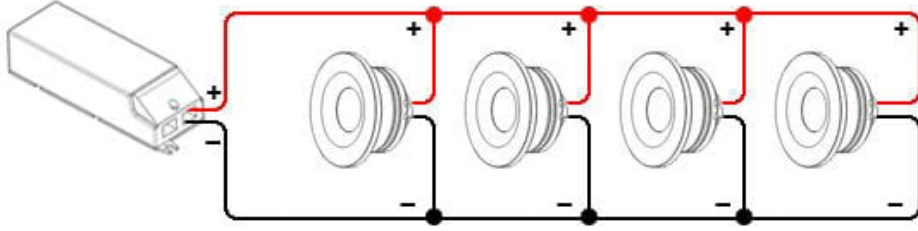
चित्र 2.3.1 (बी) 12V, 24 V, और 230V पर समानांतर कनेक्शन
